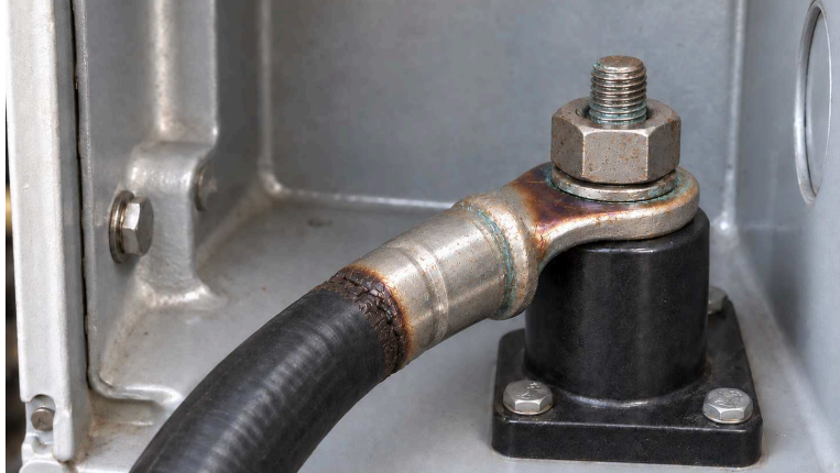
BEFORE: வெப்பத்தால் பழுதான JOINT
