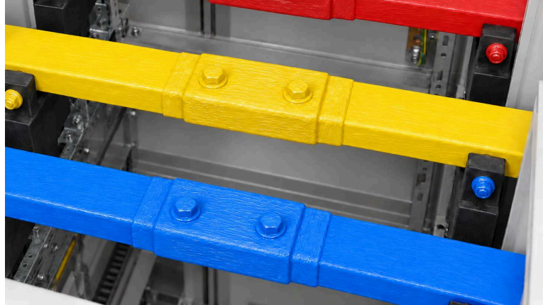
AFTER: COAT செய்த JOINT & BOLT
