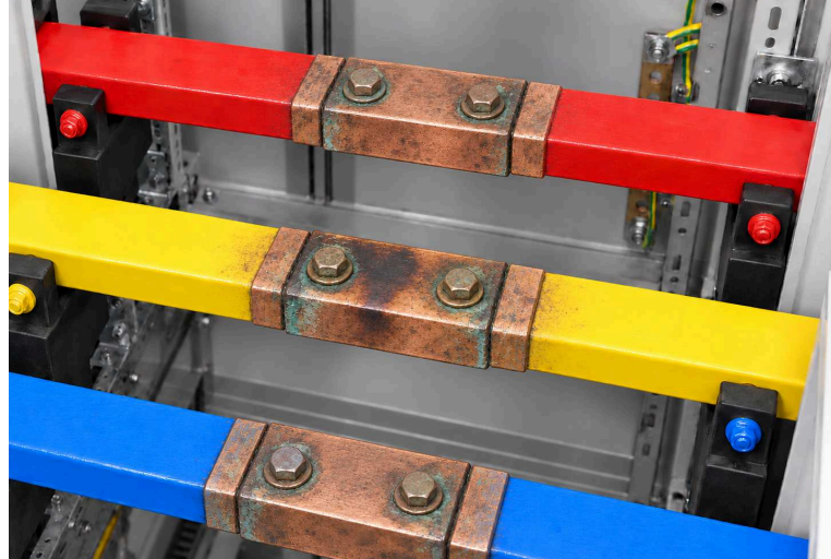
پہلے: SPLICE میں CORROSION
